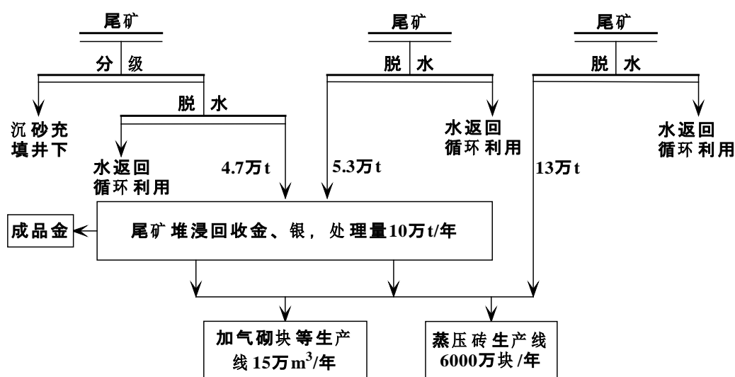
图 24 工艺流程图
