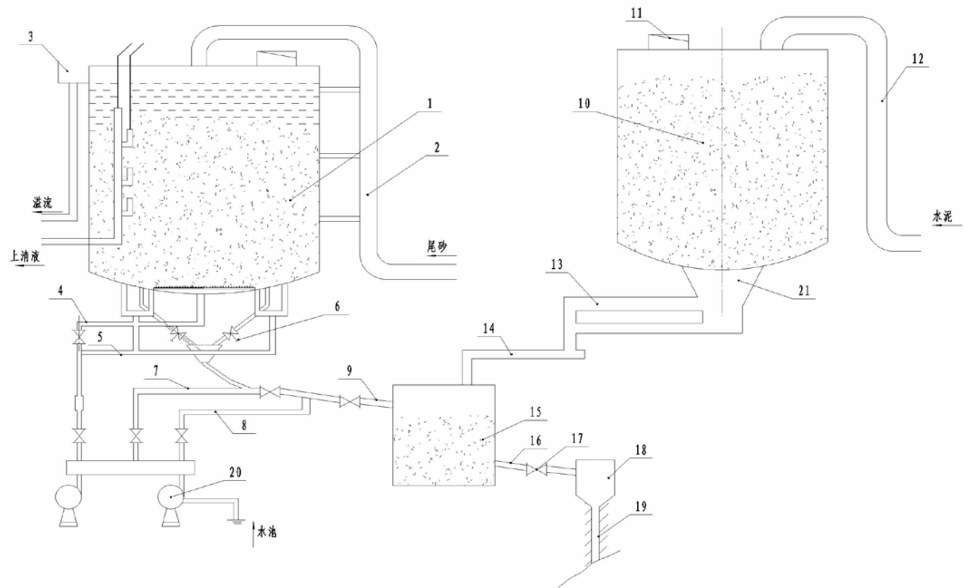
1. 立式砂仓 2. 供砂管 3. 溢流环槽及溢流管 4. 松动尾砂喷咀水管 5. 送浆喷咀水管 6. 等阻力放砂管 7. 调节浓度水管 8. 导流管 9. 下砂总管 10. 水泥仓 11. 重物物位计 12. 水泥输送管 13. 双螺旋喂料机 14. 微机螺旋定量给料称 15. 搅拌桶 16. 下浆总管 17. 电子夹管阀 18. 集浆漏斗 19. 钻孔 20. 水泵 21. 下料漏斗
