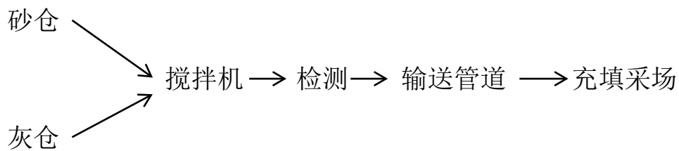
图 28 尾矿胶结充填工艺流程
