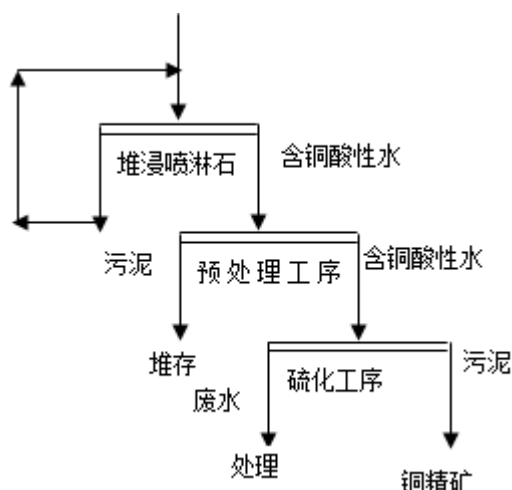
图 10 工艺流程图
