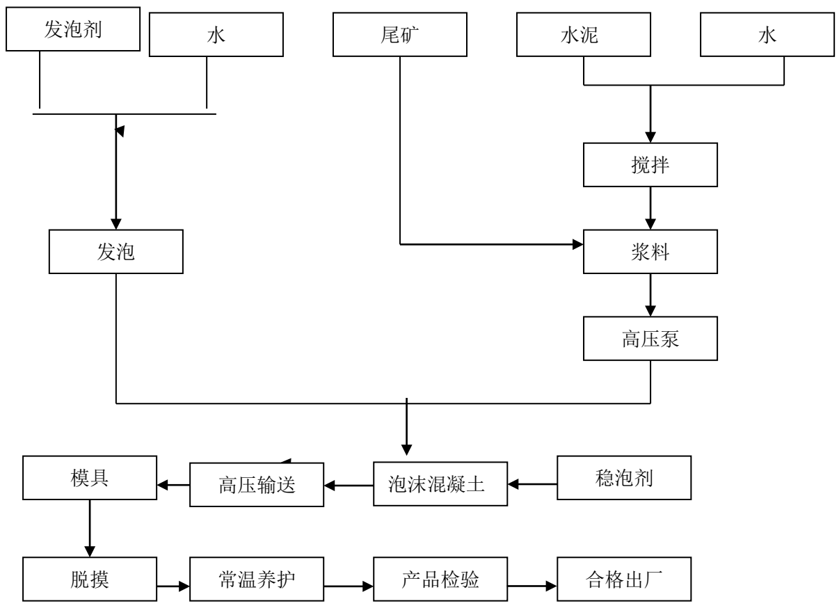
图 18 尾矿泡沫混凝土砌块规模化试生产工艺流程
