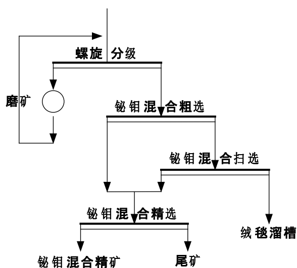
图 8 工艺流程
