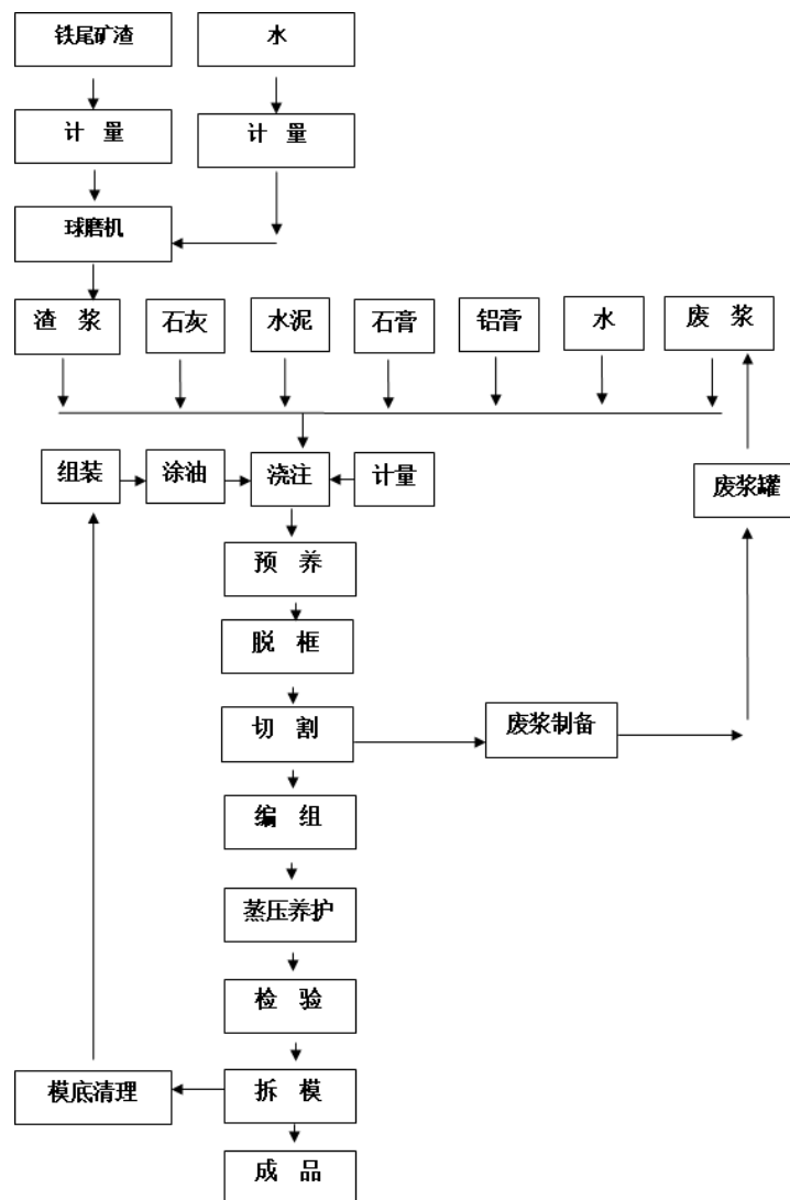
图 19 工艺流程图
