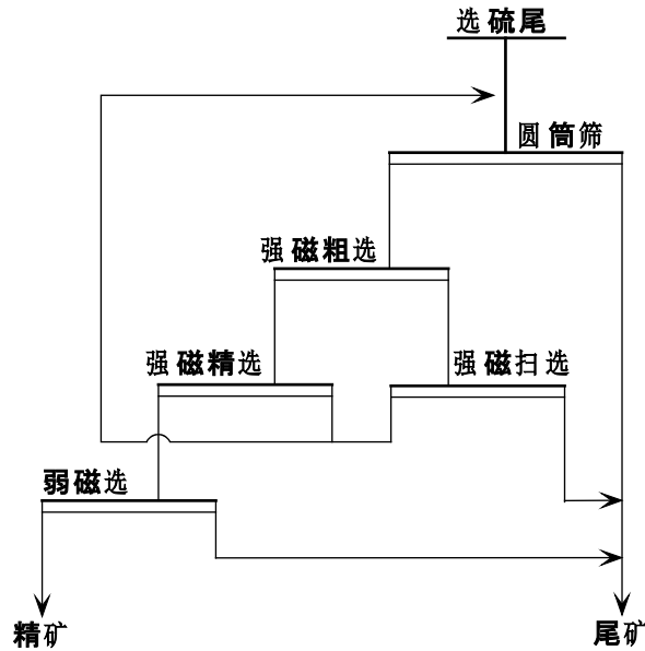
图 7 工艺流程
