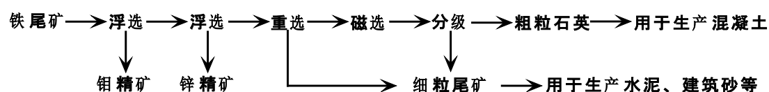
图 23 工艺流程
