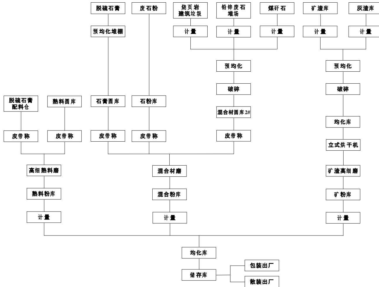
图 14 利用铅锌尾矿等工业废弃物作为混合材生产 P.C 水泥的工艺流程
