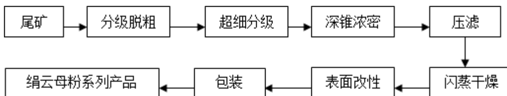
图 6 工艺流程
