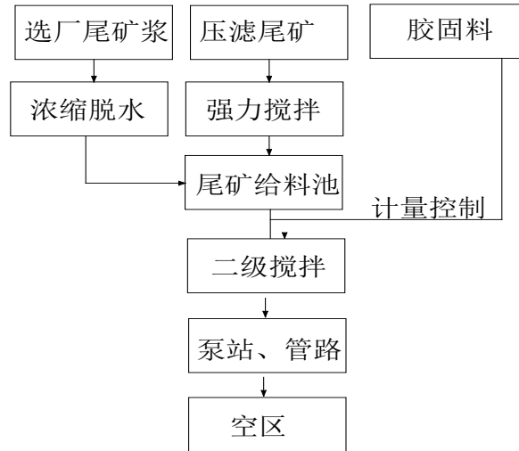
图 30 工艺流程
